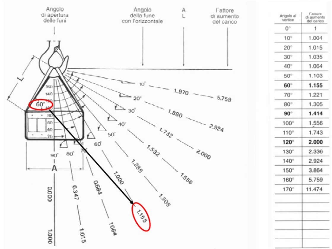
Diagramma delle portate in funzione delle variazioni dell'angolo di lavoro
