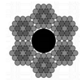
fune
