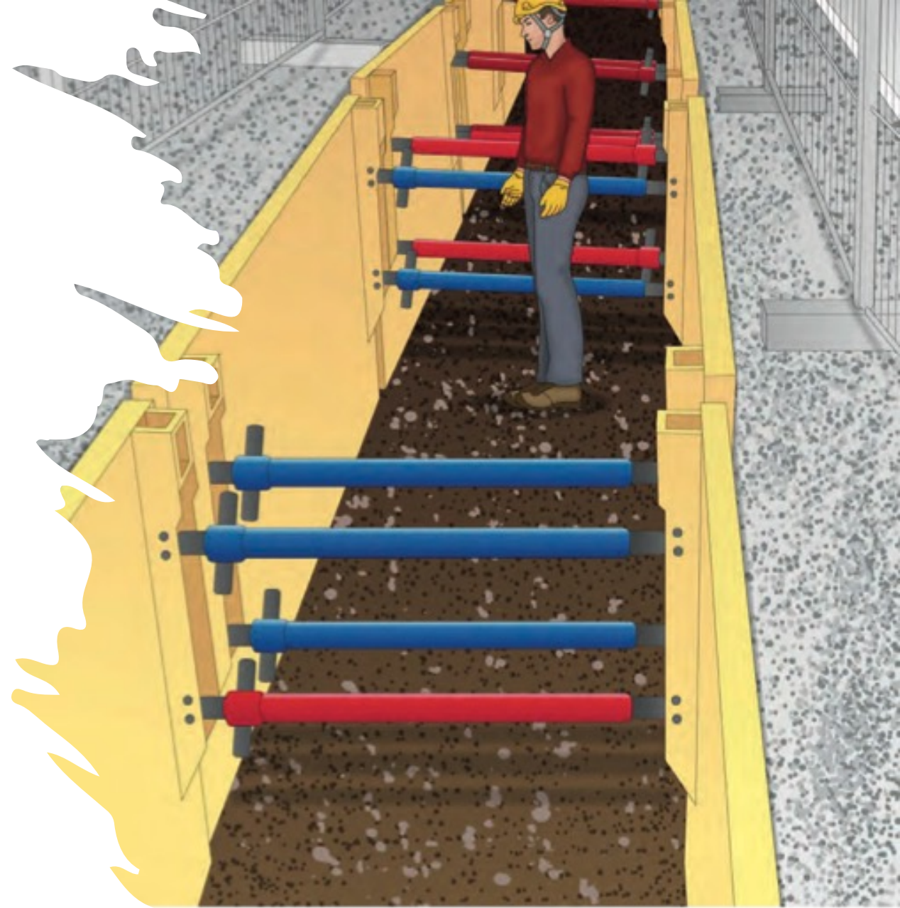
- Sistema di puntellazione per scavi supportato ai bordi con puntelli con regolazione variabile della lunghezza
