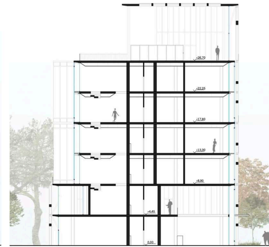
Sezione 3
